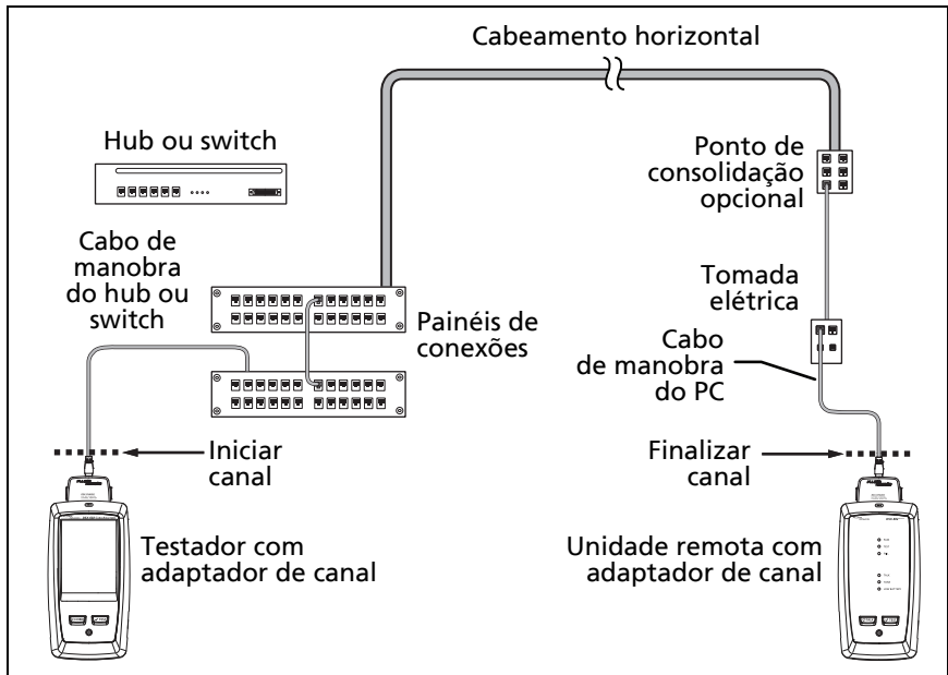
Figura 15. Conexões de canal
