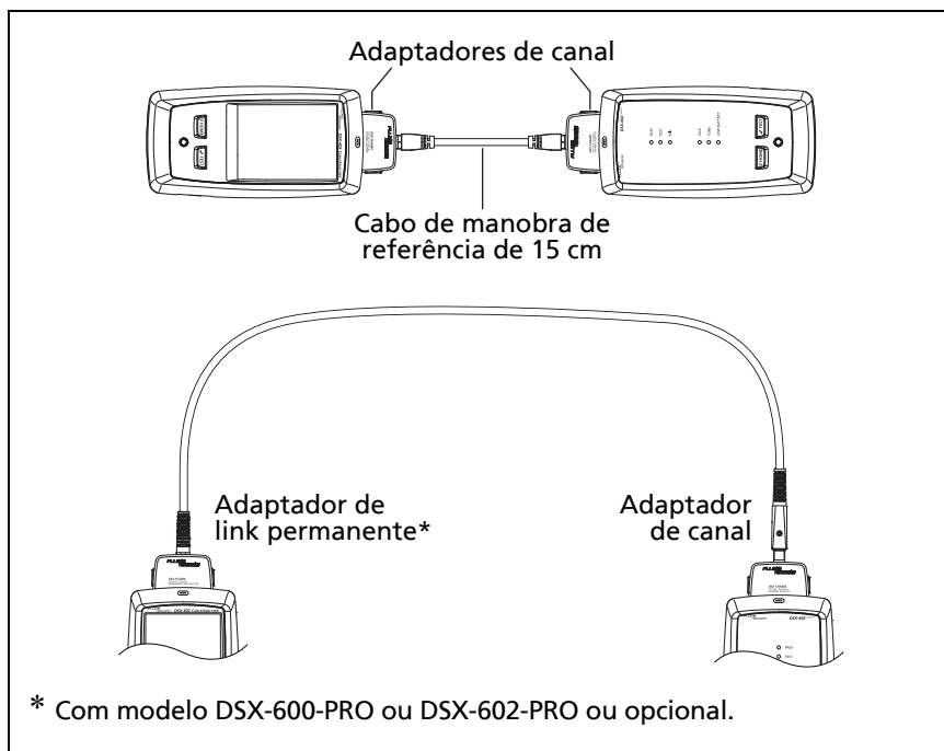
Figura 10. Conexões de referência para cabo de par trançado
