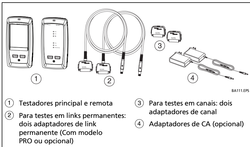
Figura 13. Equipamento para os autotestes no cabo de par trançado
