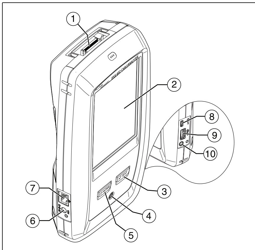
Figura 1. Conectores do testador principal, teclas e LEDs
