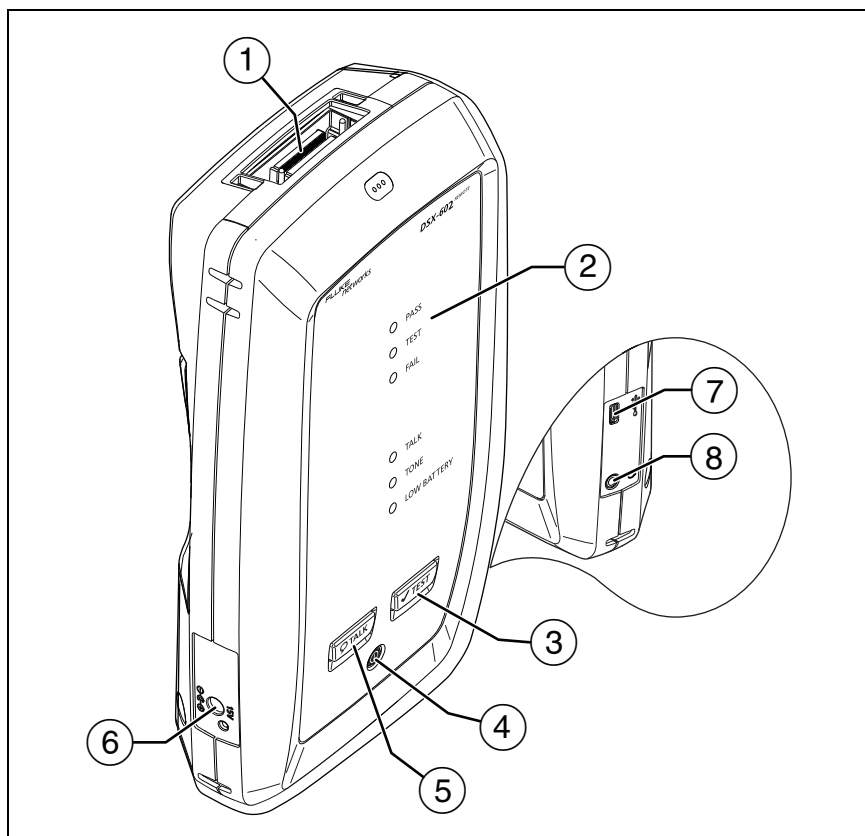
Figura 2. Conectores do testador remoto, teclas e LEDs
