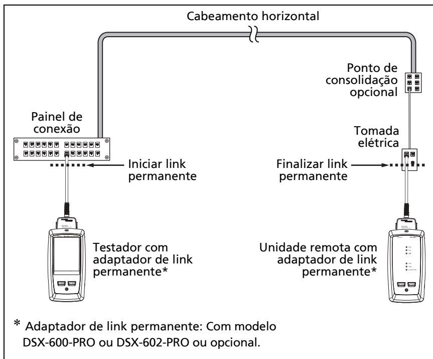
Figura 14. Conexões de link permanente
