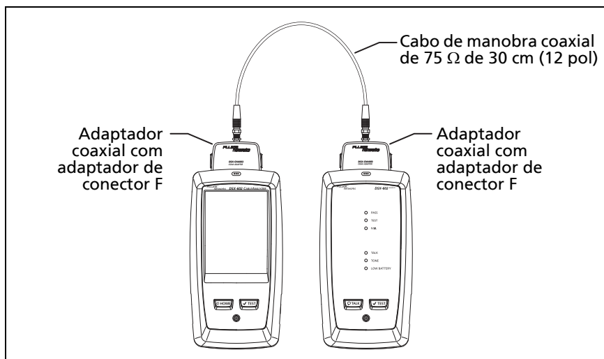
Figura 22. Conexões de referência para testes em cabeamento coaxial
