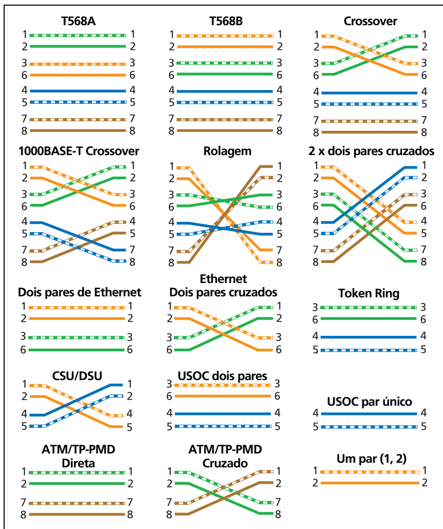
Figura 11. Configuração de tomada - RJ45
